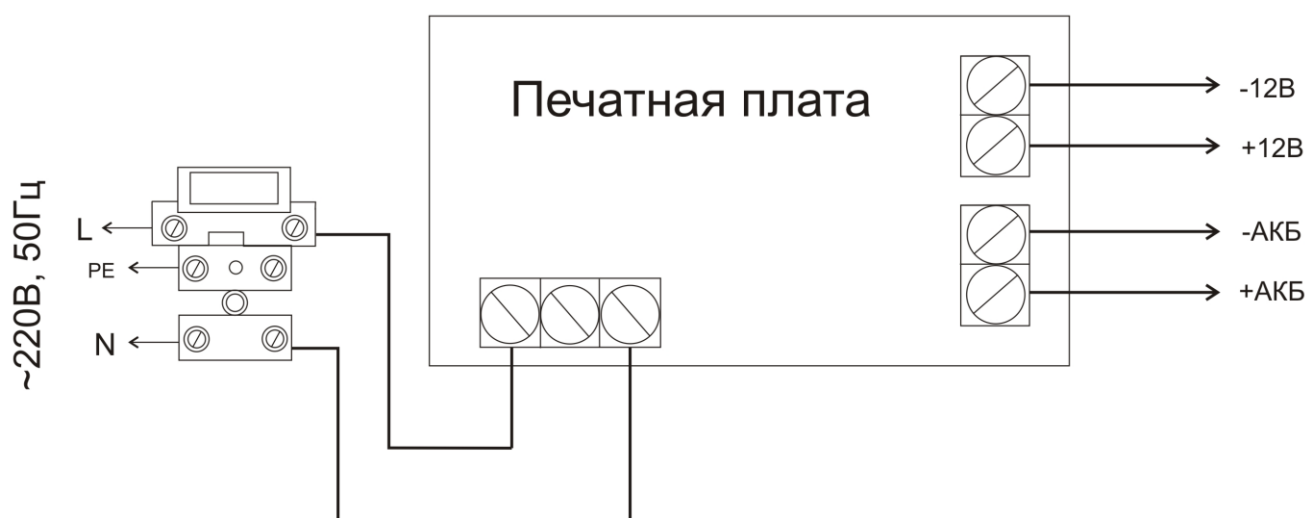
Рис. 1 Схема подключения
